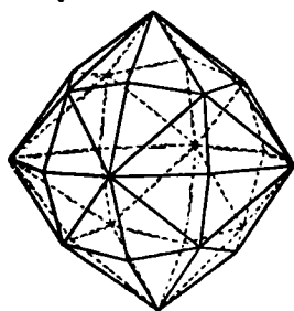
FIG. 24.—Hexakis-octahedron.
