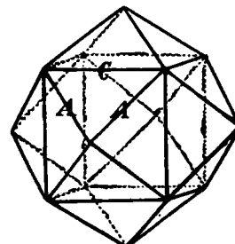
FIG. 22.—Tetrakis-hexahedron.
