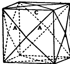
FIG. 21.—Tetrakis-hexahedron.
