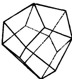
FIG. 27.—Deltoid Dodecahedron.
