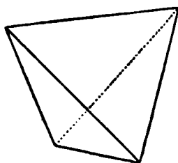
FIG. 26.—Tetrahedron.
