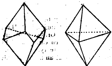
FIG. 74.—Trigonal Trapezohedron.
