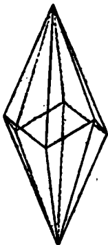
FIG. 68.—Scalenohedron.
