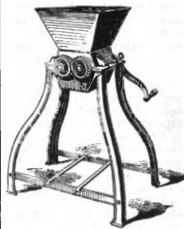
FIG. 6.—Curd-Mill.
