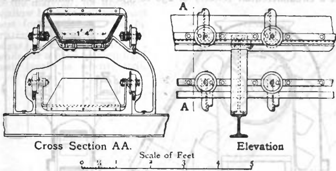
FIG. 12.—Wild Coke Conveyor.
