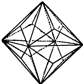
FIG. 15.—Triakis-octahedron.
