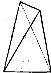
FIG. 61.—Orthorhombic Bisphenoid.
