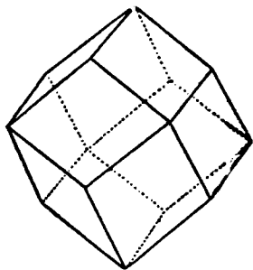
FIG. 13.—Rhombic Dodecahedron.
