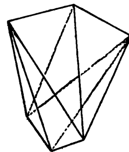
FIG. 51.—Tetragonal Scalenohedron.
