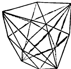
Fig. 29.—Hexakis-tetrahedron.
