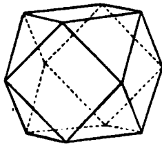
FIG. 7.—Cubo-octahedron.
