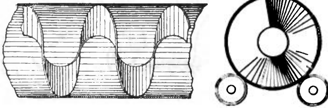
FIG. 5.—Tubular Worm Conveyor.
